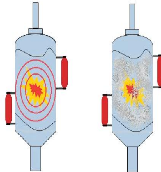
Figura 14: Sequenza di intervento dei soppressori
