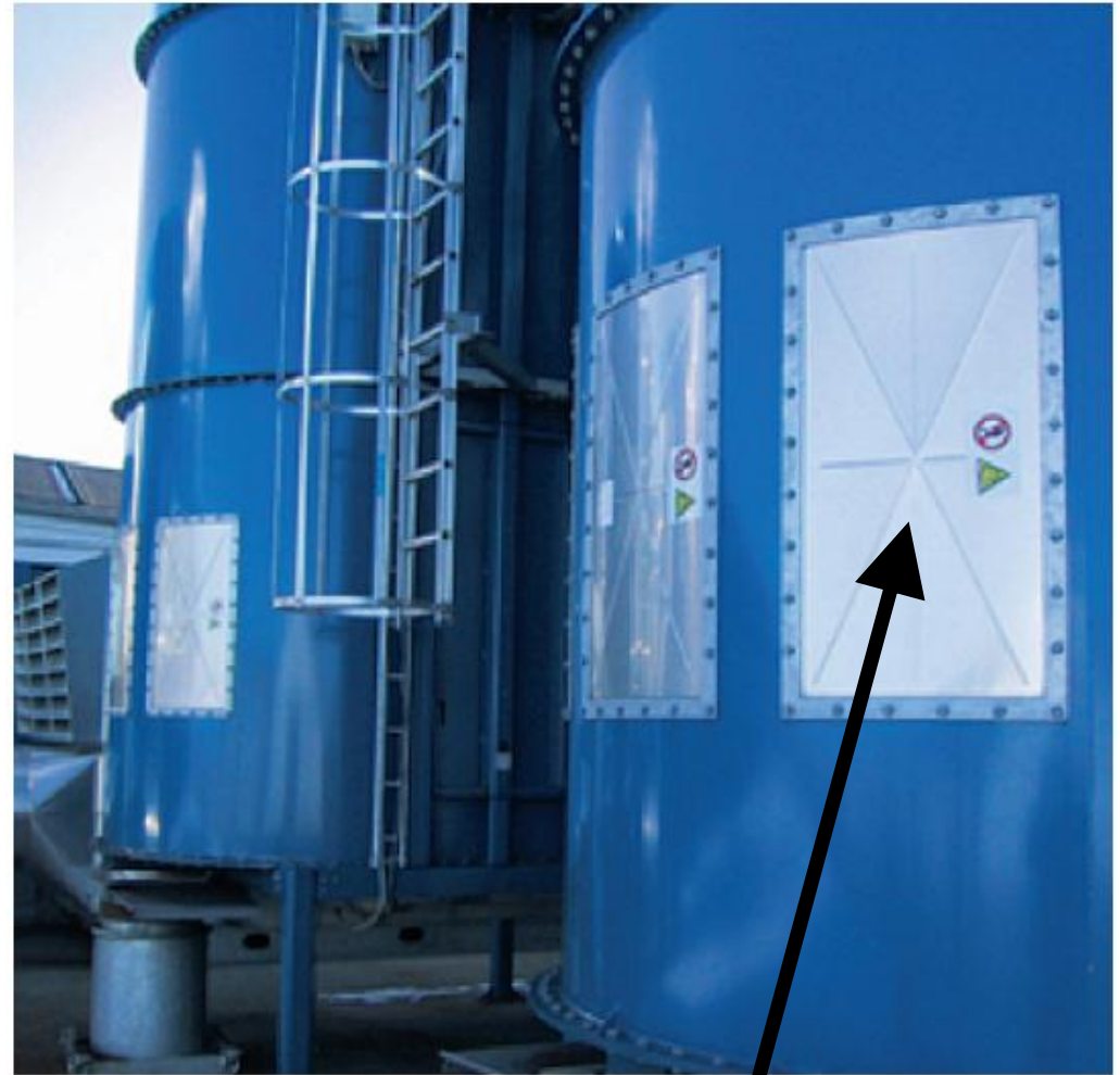
Pannelli di rottura
